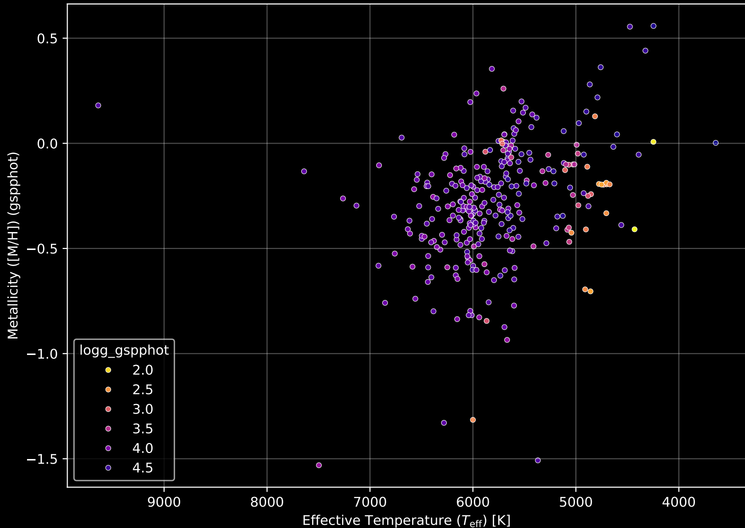
GALAH DR4 Field: [1616] Stellar Population Parameters (n= 297)
