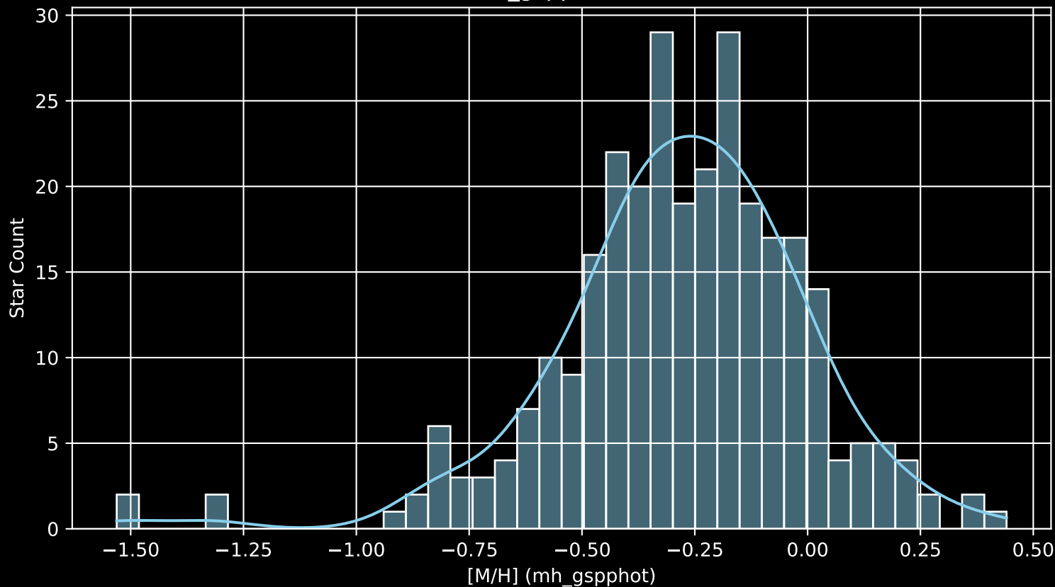
GALAH DR4 Field: [1616] [M/H] (mh_gspphot) (n= 295)
